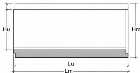
SECCION LONGITUDINAL 1/20
