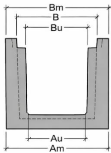
SECCION TRANSVERSAL 1/20
