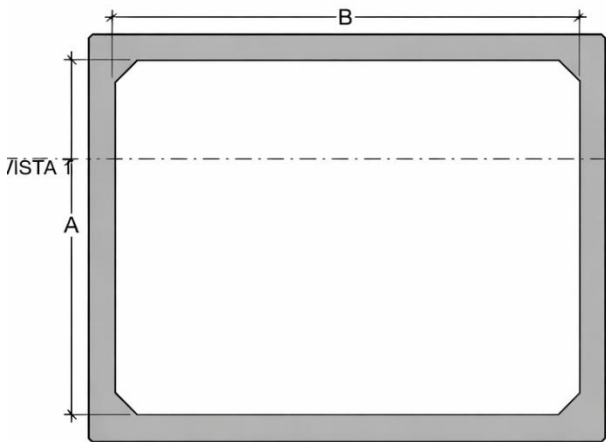
PLANTA 1/40
