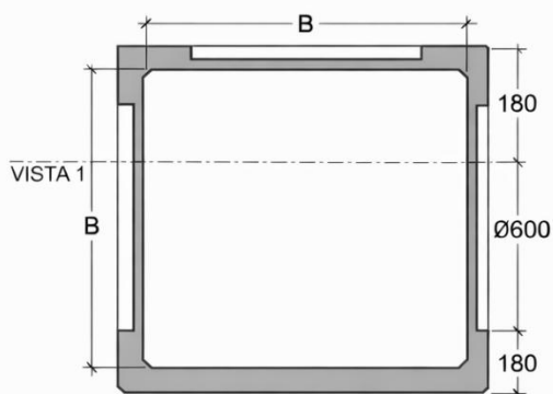
PLANTA 1/20
